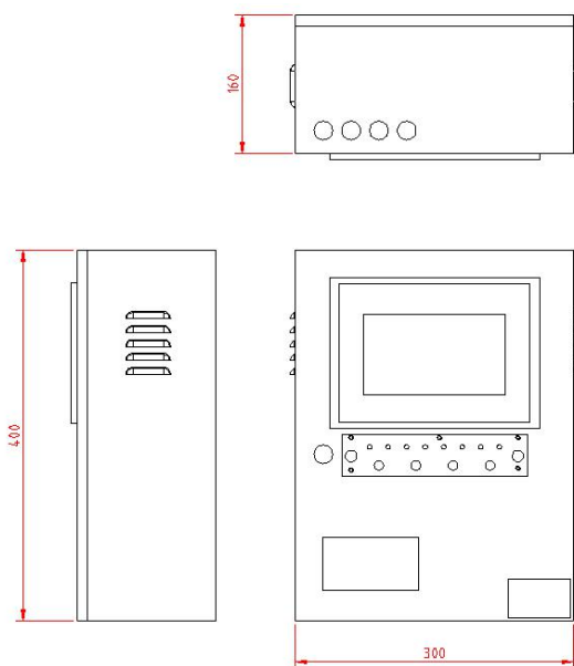
图3 AFPM100/B3 消防设备电源状态监控器外形尺寸
