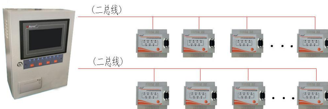
图 2 系统示意图
