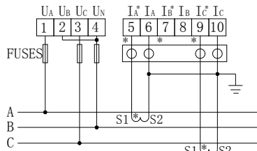
三相三线2CT
