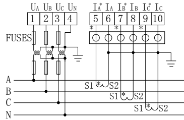
三相四线3PT、3CT
