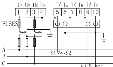
三相三线2PT、2CT
