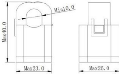
Φ 10mm
