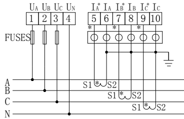
三相四线3CT
